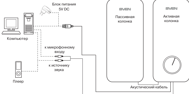
Рис. 2. Схема подключения
